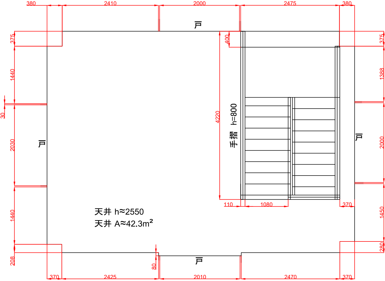
天守閣 平面図 S=1:50
